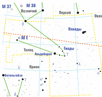
Расположение Крабовидной туманности в созвездии Тельца
